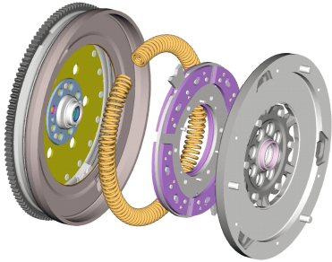
Volante bimasa
