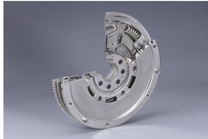
Volante bimasa
